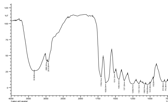
Gambar 4. Spektrum FTIR ekstrak etil asetat
