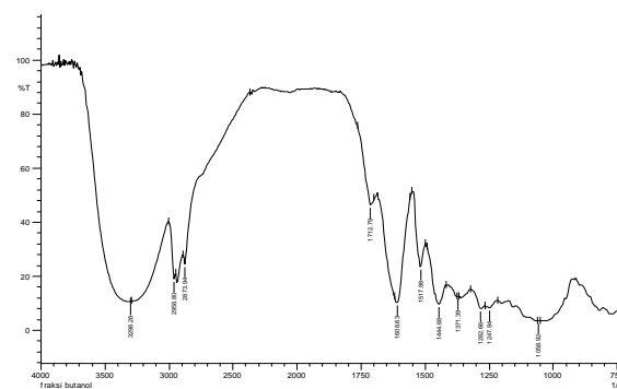
Gambar 5. Spektrum FTIR ekstrak n-butanol
